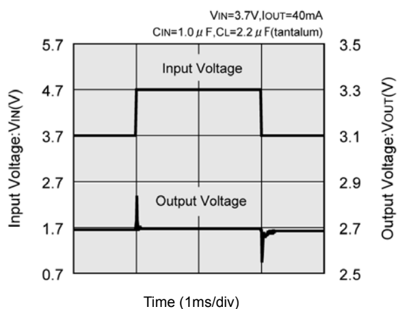
XC6201P272
