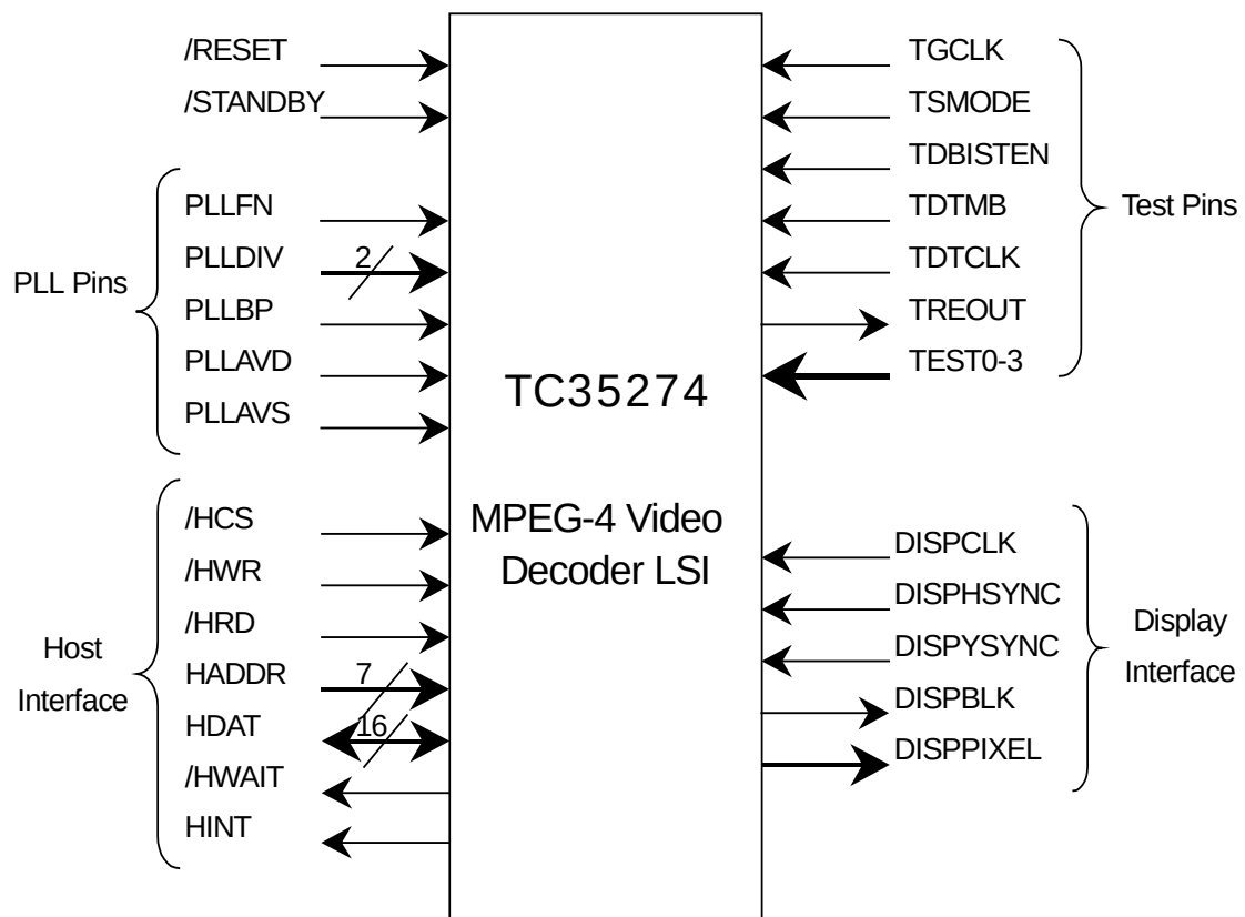
Fig. 2 Pin Map
