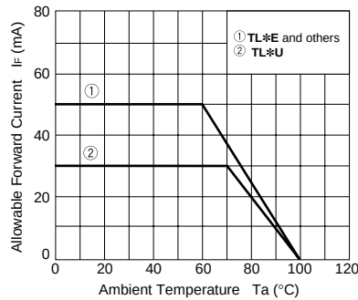
I_f - T_a
