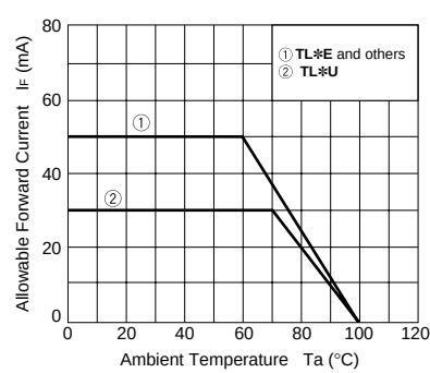
I_F - T_a
