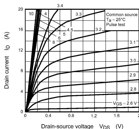
Fig. 8.2 I_D - V_{DS}
